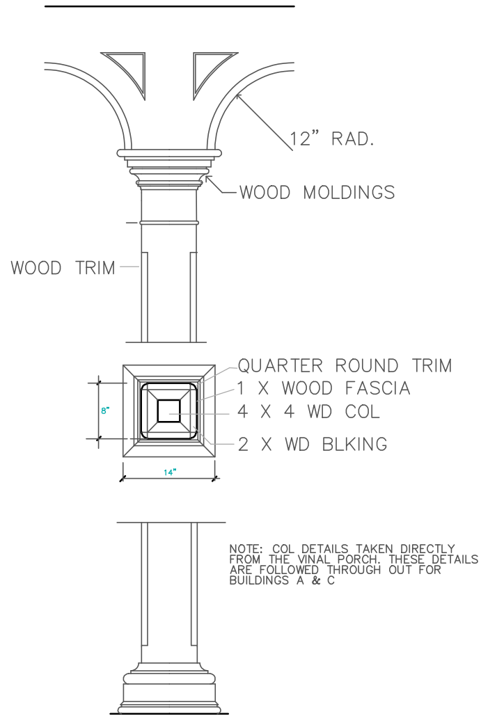
VINALE HOUSE PORCH ITALIANATE COLUMN
